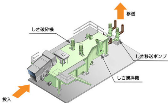
構造概念図
